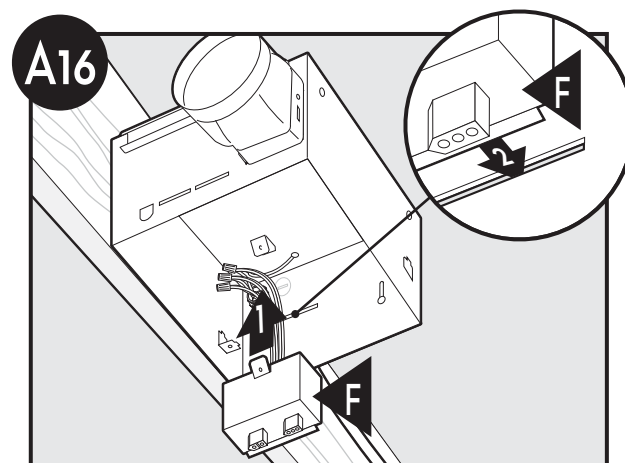
A16 Instale la placa de cubierta del cableado. Asegúrese que todas las conexiones de cableado estén dentro de la caja o debajo de la placa de cubierta del cableado.
