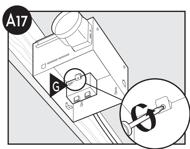
A17 Apriete el tornillo de la placa de cubierta del cableado.
