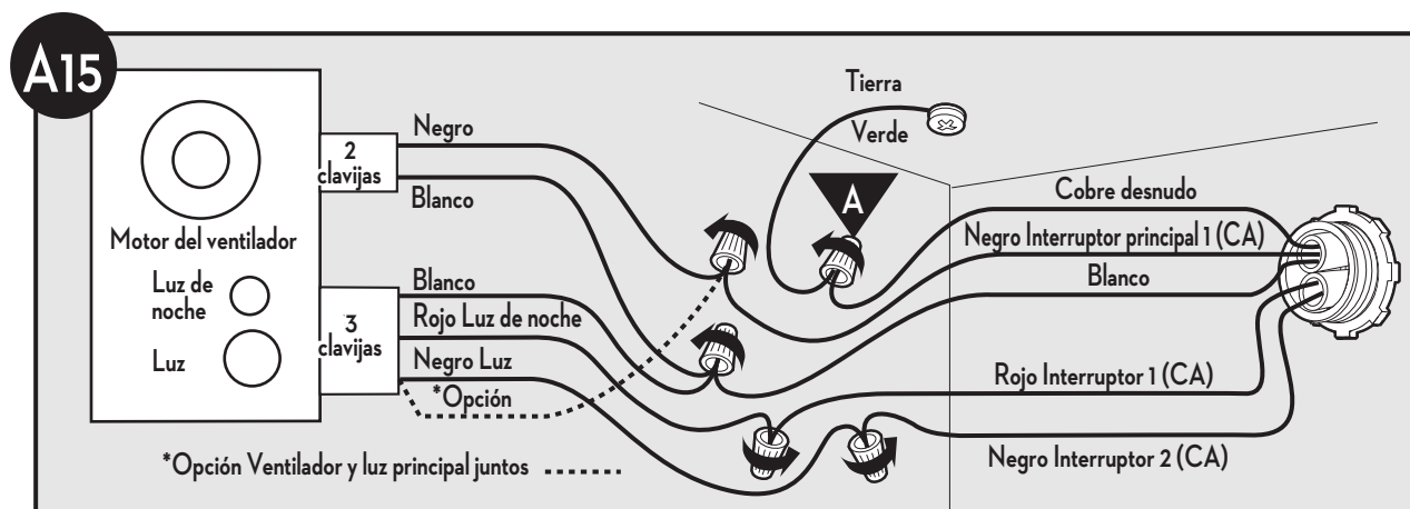
A15 Conecte los alambres como se muestra.
