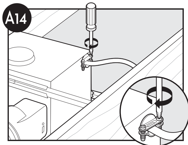
A14 Apriete los tornillos del aliviador de tensiones.
